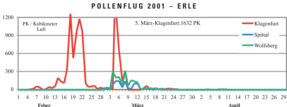
Abb. 2: Vergleichskurven des Pollenfluges der Erle ( Alnus sp. ) im Jahr 2001
