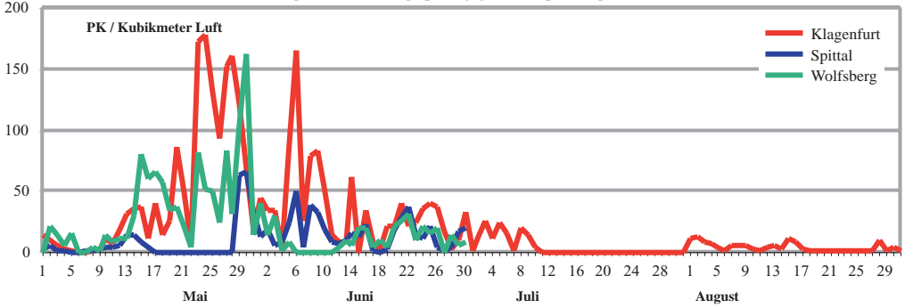
Abb. 9: Vergleichskurven des Pollenfluges der Gräser (Poaceae) im Jahr 2001
