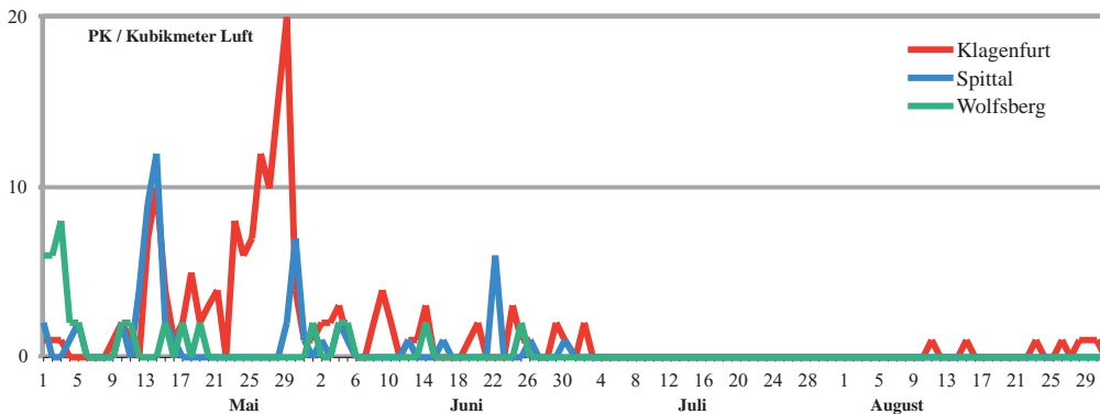
Abb. 11: Vergleichskurven des Pollenfluges des Ampfers ( Rumex sp. ) im Jahr 2001
