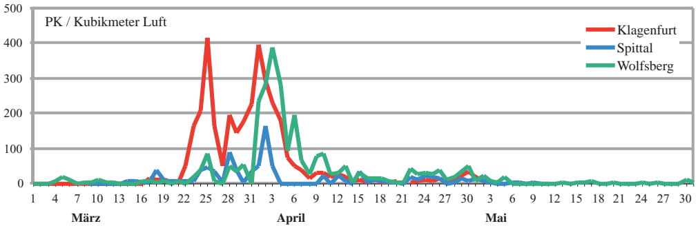
Abb. 5: Vergleichskurven des Pollenfluges der Esche ( Fraxinus excelsior ) im Jahr 2001
