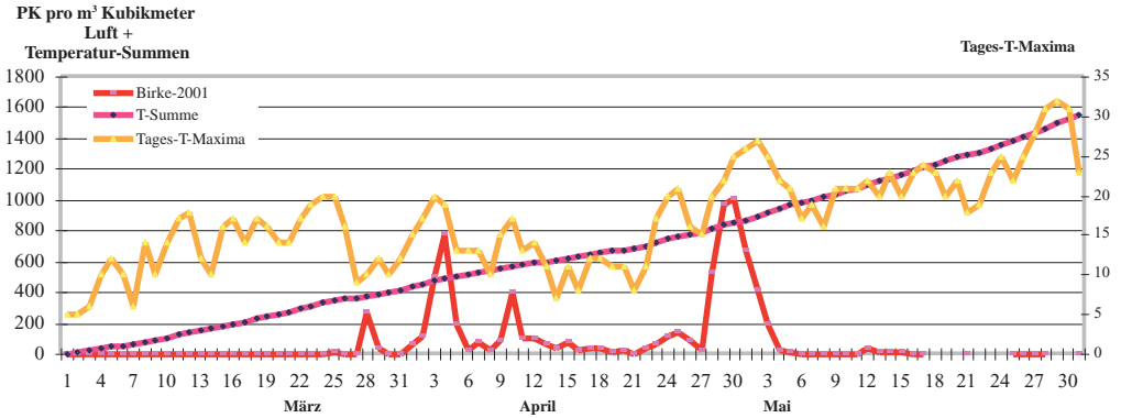
Abb. 7: Zusammenhang zwischen dem Pollenflug der Birke ( Betula pendula ) und den Temperatur-Verhältnissen in Klagenfurt im Jahr 2001
