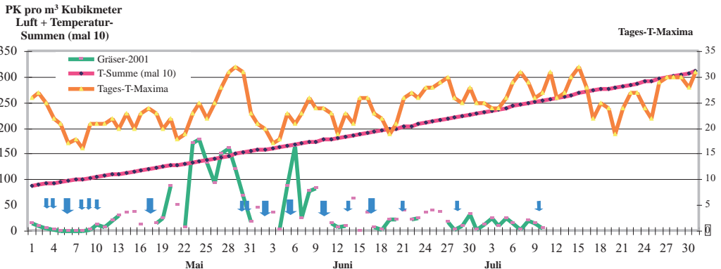
Abb. 10: Zusammenhang zwischen dem Pollenflug der Gräser (Poaceae), der Temperatur und den Niederschlagsverhältnissen im Jahr 2001
