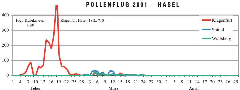
Abb. 3: Vergleichskurven des Pollenfluges der Hasel ( Corylus avellana ) im Jahr 2001
